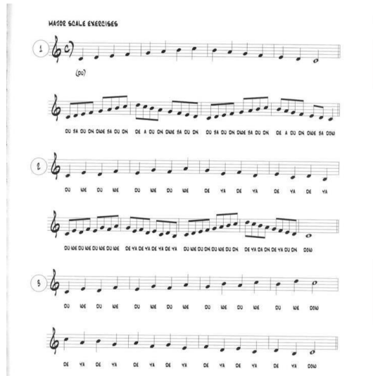
Gambar 2.1 Part Vokalisasi
